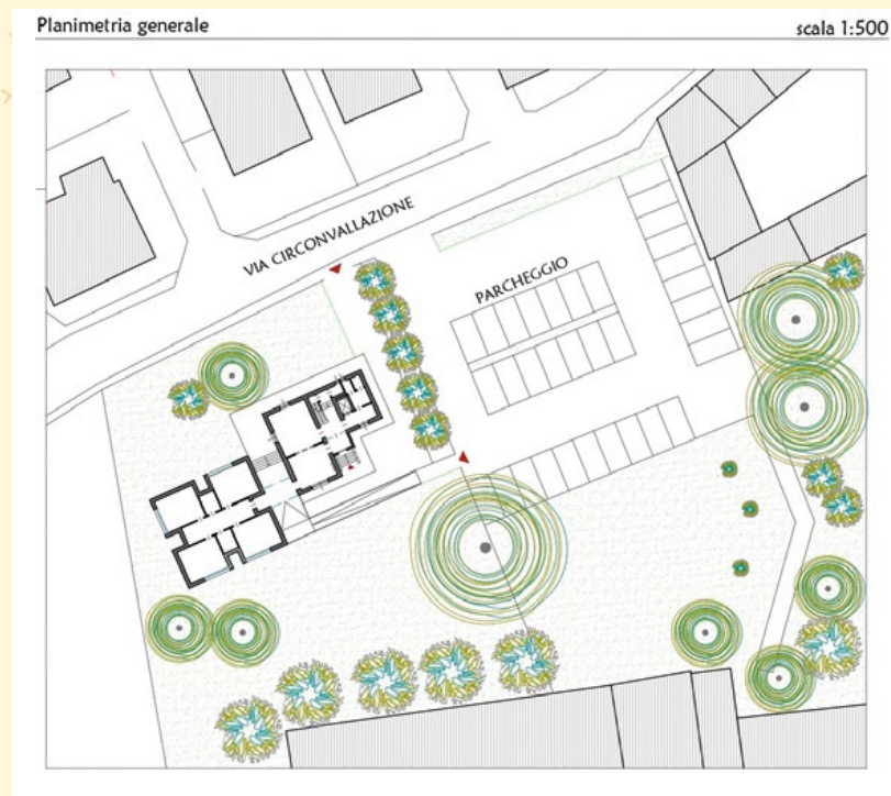
Il progetto della struttura poliambulatoriale di Via Circonvallazione
