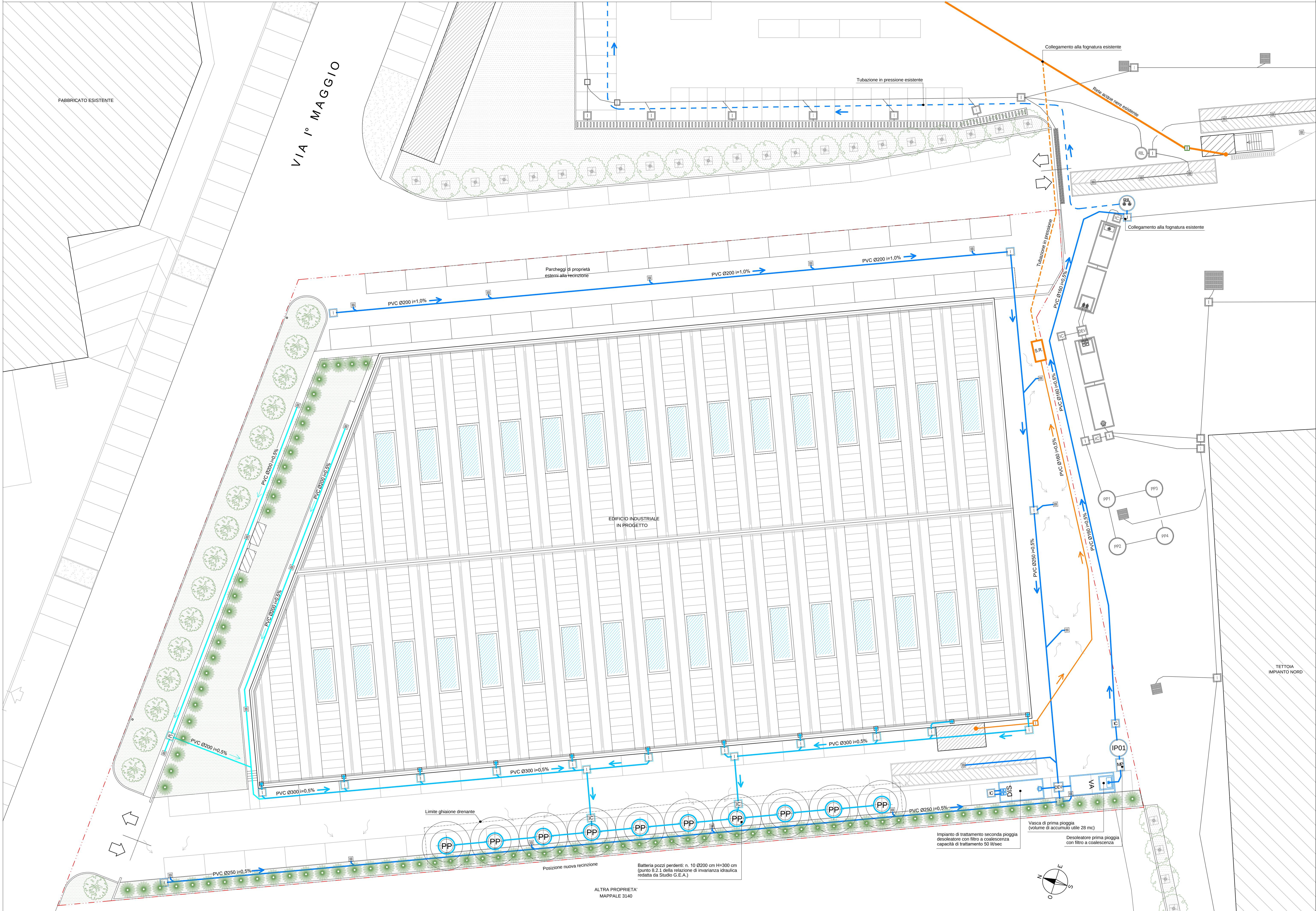
Schema Impianto Fognario - Planimetria copertura
