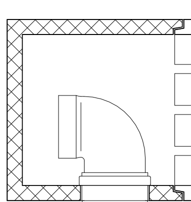
Q.S. 50X50 SEZIONE
