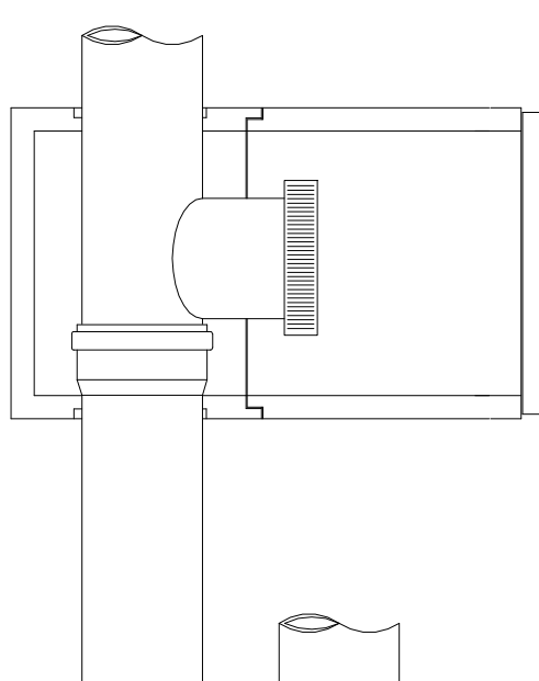
Q.S. 40X40 EQUIVALENTE CON PROLUNGA SEZIONE
