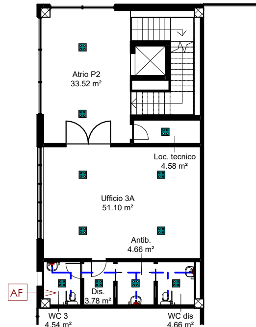
Pianta piano primo - Porzione A | scala 1:200
